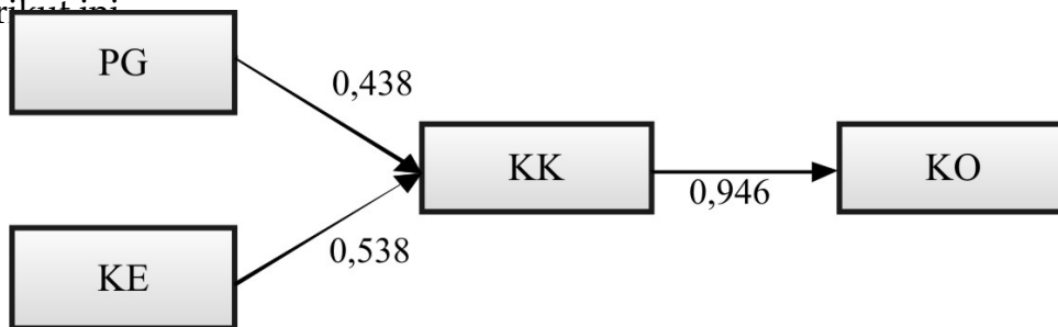
Gambar 4 Path Analysis Peran Ganda, Kelelahan Emosional, Kepuasan Kerja dan Komitmen Organisasi
