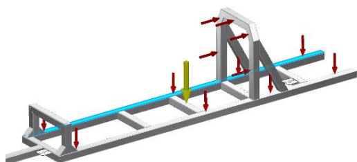
Gambar 3. Beban yang diterima dudukan roda depan kanan
