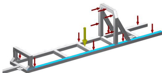
Gambar 4. Beban yang diterima dudukan roda depan kiri
