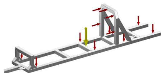
Gambar 1. Arah gaya yang diterima struktur rangka sasis
