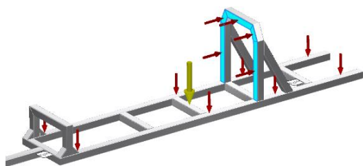
Gambar 2. Beban yang diterima roll bar pengemudi
