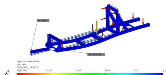
Gambar 5. Von Mises Stress
