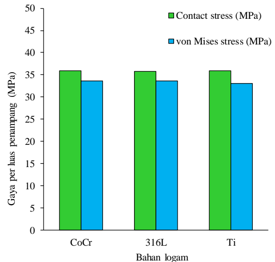
Gambar 8. Luaran besaran tekanan kontak dan tegangan kerja pada bahan UHMWPE untuk beban panggul.
