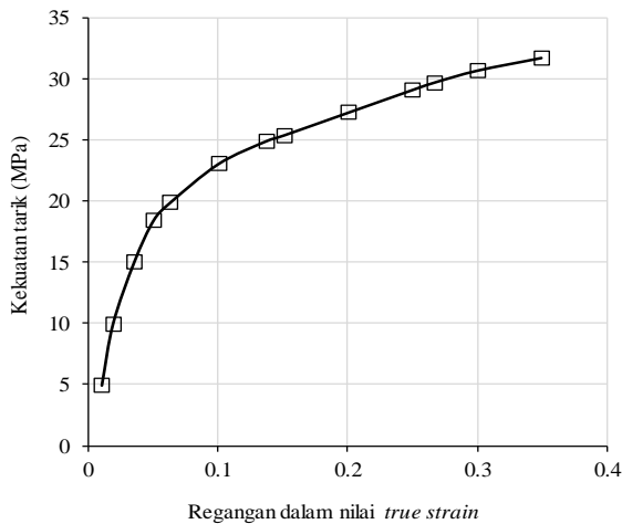
Gambar 4. Model material UHMWPE menurut Kang dkk. (Kang, et al., 2017)
