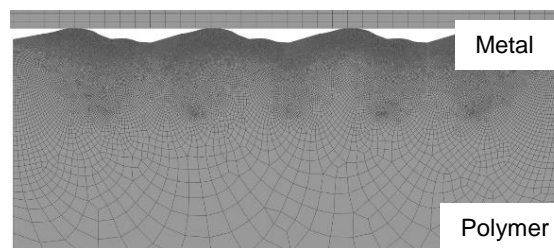
Gambar 3. Model CAE asperity permukaan UHMWPE hasil pemesinan
