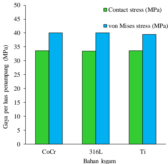
Gambar 7. Luaran besaran tekanan kontak dan tegangan kerja yang diderita bahan UHMWPE untuk beban lutut
