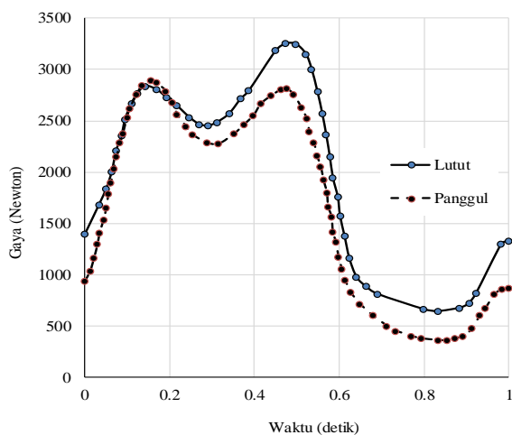
Gambar 5. Siklus beban panggul (Bergmann, Bender, Dymke, Duda, & Damm, 2016) dan lutut (Bergmann, et al., 2014)
