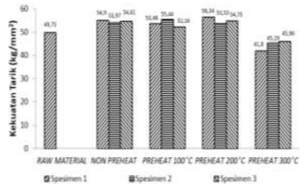
Gambar 17. Histogram Hasil Pengujian Tarik
