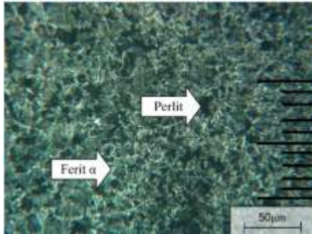
Gambar 10). HAZ preheat 100 0 C
