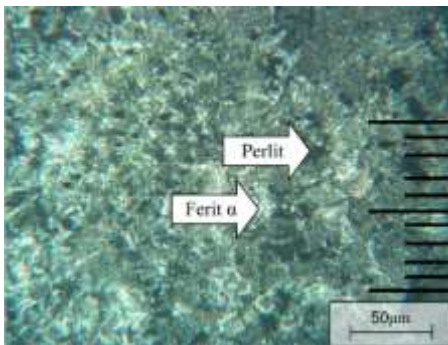
Gambar 12). HAZ preheat 300 0 C
